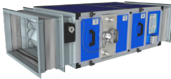
Установка SEZON MB15 R W2 *Длина указана без учета гибких вставок (80-140 мм каждая) и воздушного клапана (125 мм).
